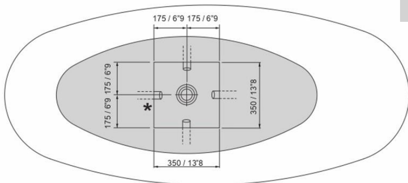
Area della base della vasca
